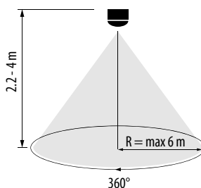
Височина на инсталиране: 2.2 - 4 m
