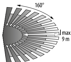
Обхват на действие: 160°, max. 9m
