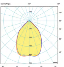
Светлоразпределителна диаграма с дифузер 80° (LSFL80)
