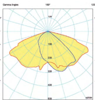
Светлоразпределение: 90°x140° (Type III по IESNA)
