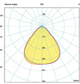
Светлоразпределителна диаграма с дифузер 90° (LIK190)
