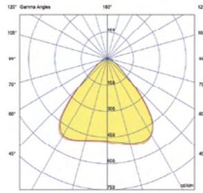
Светлоразпределителна диаграма с дифузер 90° (LIK15090)
