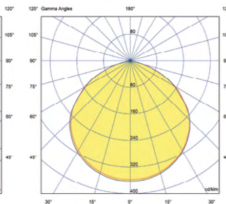
Светлоразпределителна диаграма с дифузер 110° за модели LSF20050D110, LSF15050D110, LSF10050D110
