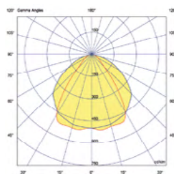
Светлоразпределителна диаграма с дифузер 90°x110° (LDH90110)
