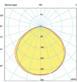
Светлоразпределителна диаграма с дифузер 120° (LIK120)
