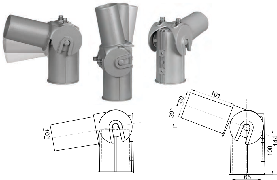
АДАПТЕР Ø60 MM С РЕГУЛИРАНЕ ЪГЪЛА НА МОНТАЖ ЗА СВЕТОДИОДНИ УЛИЧНИ ТЕЛА LUT2042, LUT4042, LUT6042
