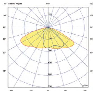
Светлоразпределение: 90°x140° (Type III по IESNA)
