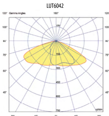
LUT6042
