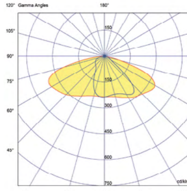
Светлоразпределение: 90°x140° (Type III по IESNA)
