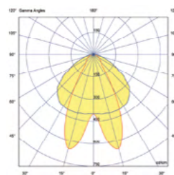
Светлоразпределителна диаграма с дифузер 2x25° (LDH25DA)
