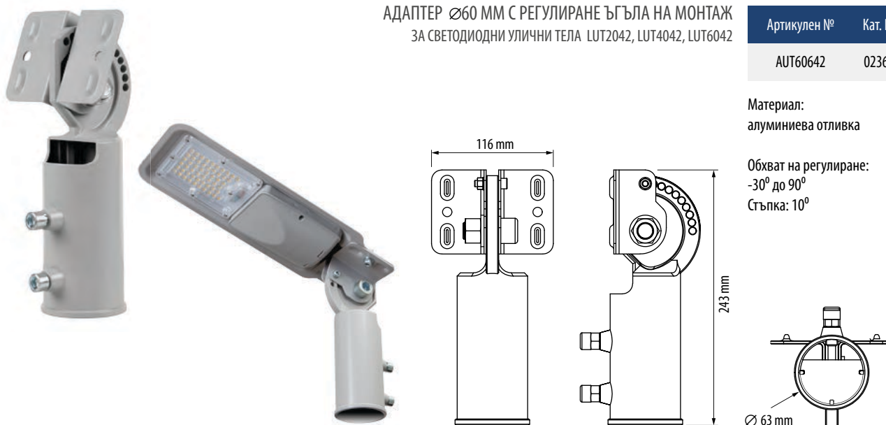
АДАПТЕР Ø60 MM С РЕГУЛИРАНЕ ЪГЪЛА НА МОНТАЖ ЗА СВЕТОДИОДНО УЛИЧНО ТЯЛО LUT10042
