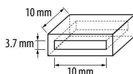
СИЛИКОНОВА ТАПА ЗА СВЕТОДИОДНА ЛЕНТА IP67 10 mm, 10 бр.
